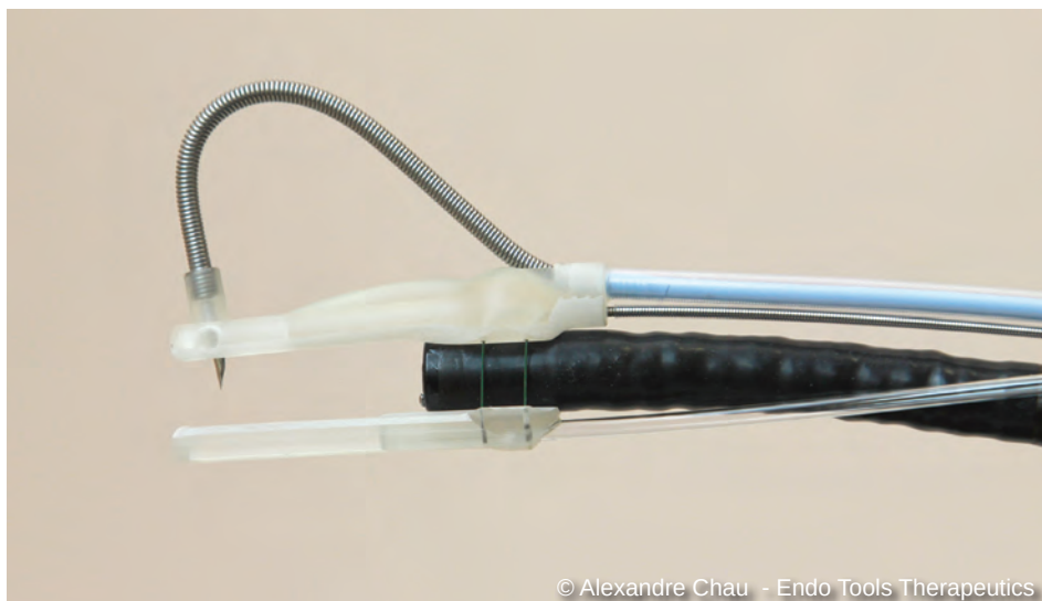
La plateforme Endomina™ montée sur un endoscope, prête à être utilisée
